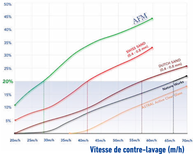
Expansion du lit filtrant à 25 °C
