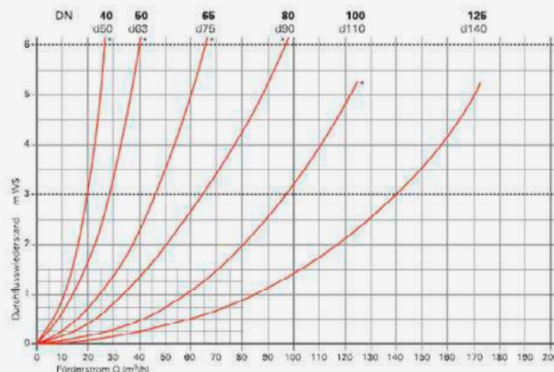
Vannes automatiques - Courbe de pertes de charge
